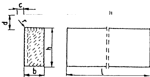
Rys. 1. Wymiarowanie krawężników
