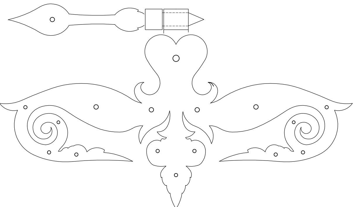
hak i zawias typ E4
