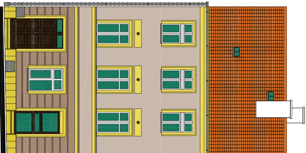
ELEWACJA POŁUDNIOWA
